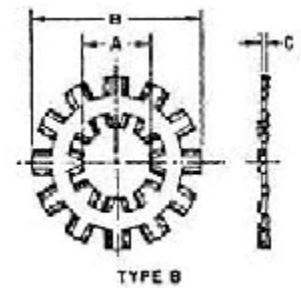
图18美国标准的内部至外部的 齿锁垫圈(ASA B27.1-1965), 类型B
