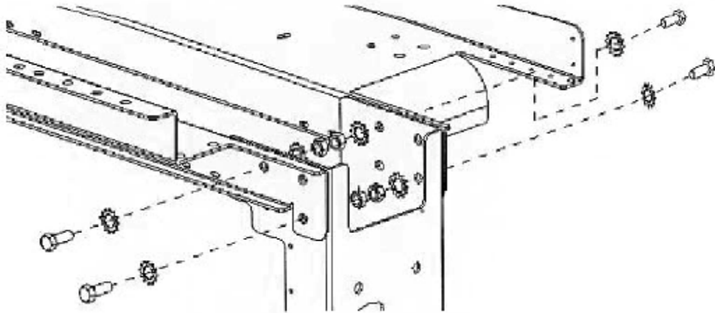
图19 典型的机柜组合硬件
